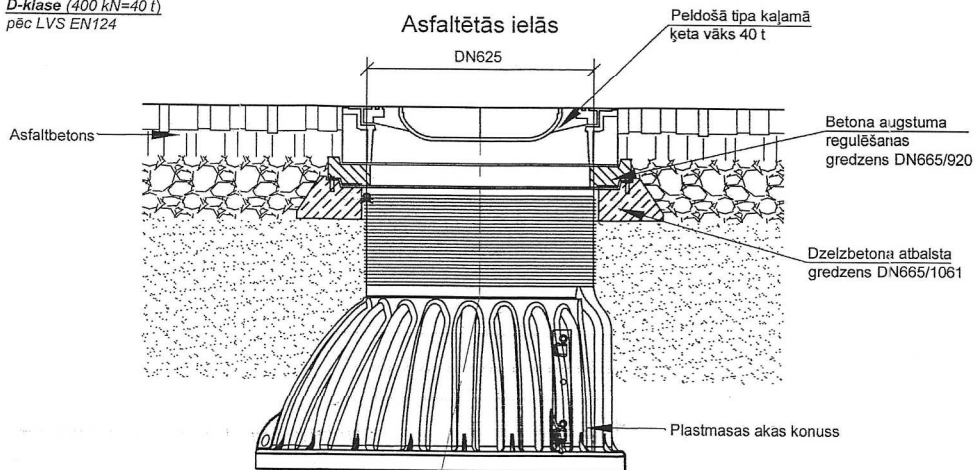
D-klase (400 kN=40 t) pēc LVS EN124
