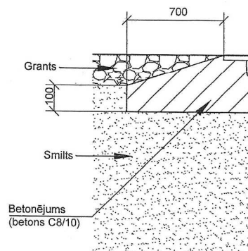
D-klase (400 kN=40 t) pēc LVS EN124
