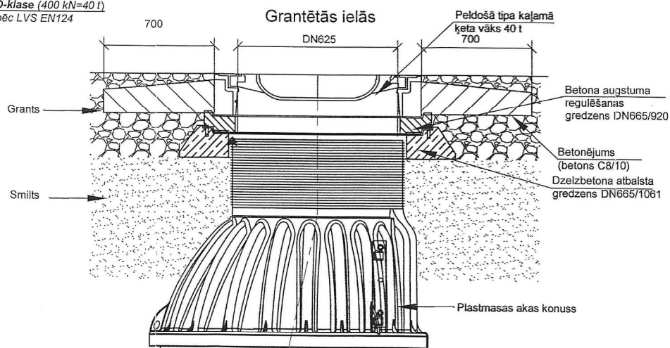
D-klase (400 kN=40 t) pēc LVS EN124
