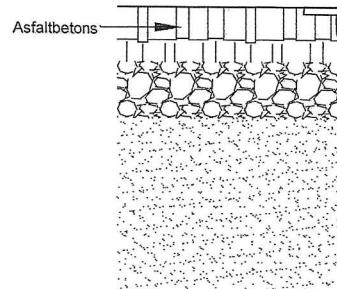
D-klase (400 kN=40 t) pēc LVS EN124
