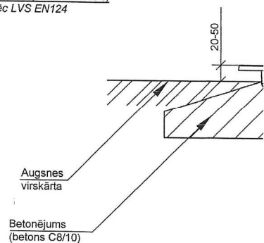
B-klase (125 kN=12.5 t) pēc LVS EN124
